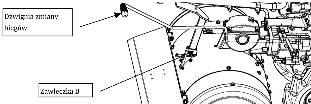
8 rys : Montaż dźwigni zmiany biegów
