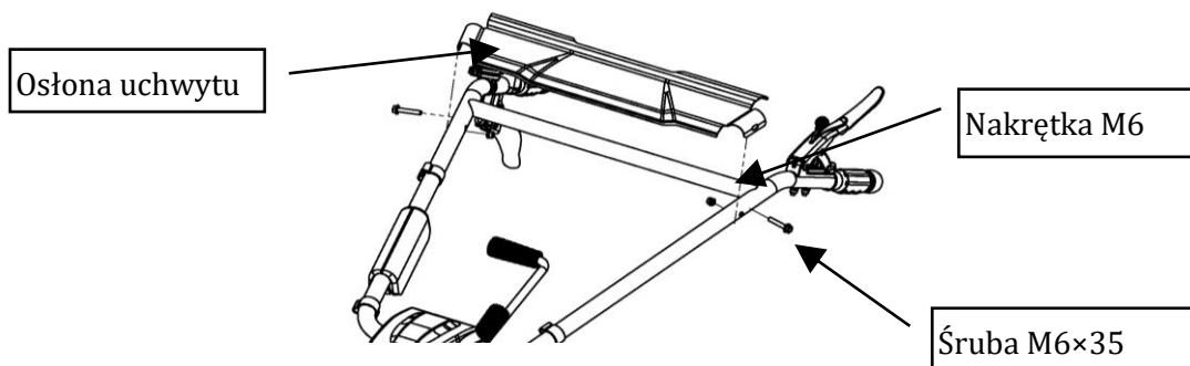
10 rys : Montaż osłony górnej
